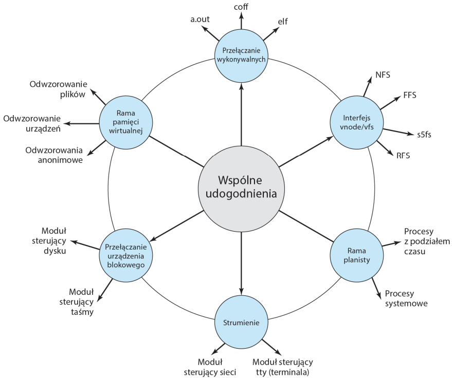
Rysunek 2.16. Jądro nowoczesnego UNIX-a
