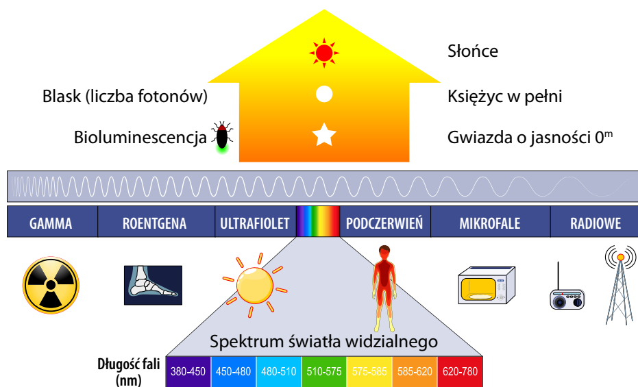
ILUSTRACJA 78. Spektrum światła
